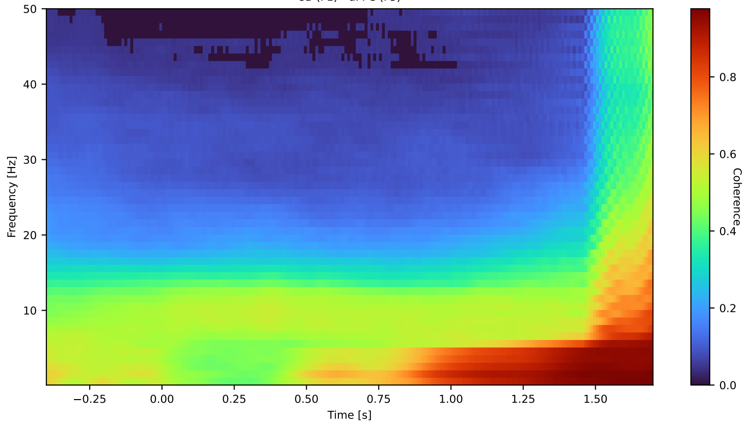
8B (F1) - dPFC (F5)
